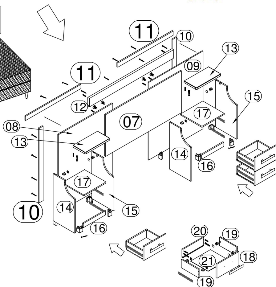
DETALHE DE GAVETA
